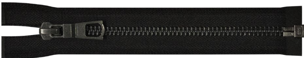
Metálico No.5 Separable, Negro Quemado Deslizador Ahumado con seguro automático
