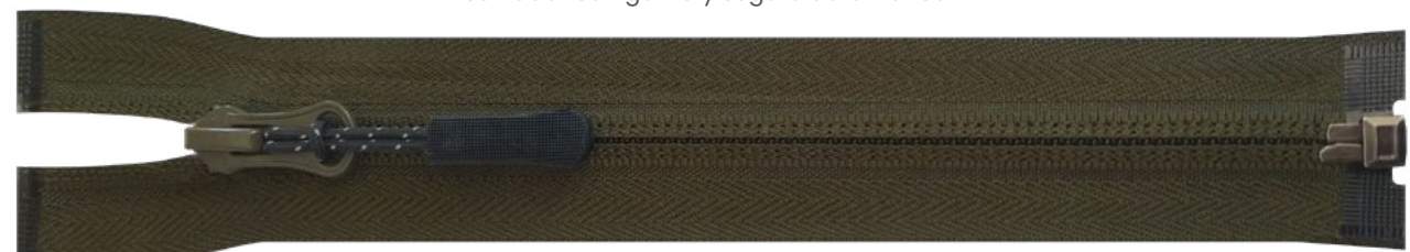
Nylon No.5 invertido, Separable Deslizador al tono con seguro automático
