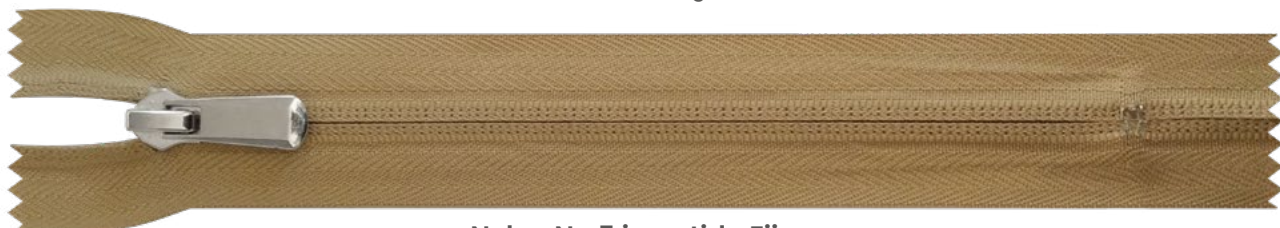
Nylon No.5 invertido,Fijo Deslizador Nickel con seguro automático
